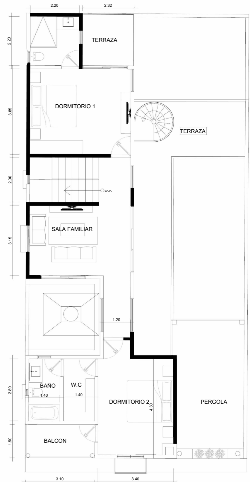
PLANTA NIVEL 2
